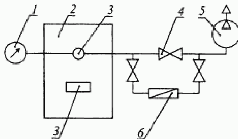
1 — микроманометр; 2 — камин; 3 — манжета резиновая; 4 — кран проходной; 5 — вакуум-насос; 6 — расходомер
